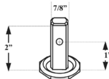
-42- OCTAGON STEM
