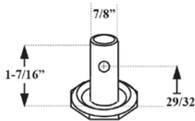
-31- ROUND STEM
